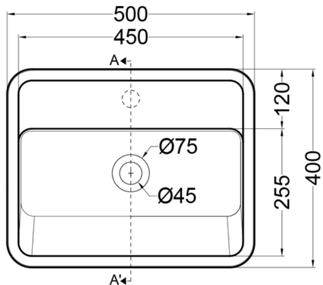
PIANTA
