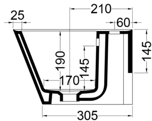
SEZIONE A-A'
