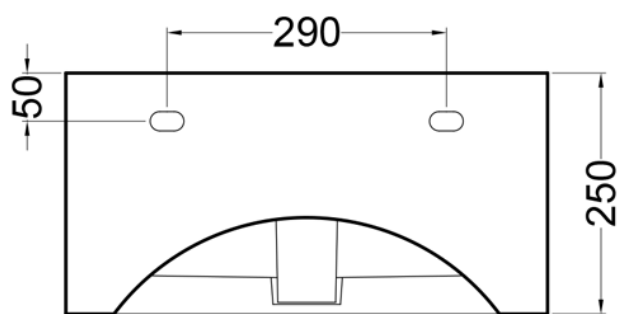
VISTA POSTERIORE
