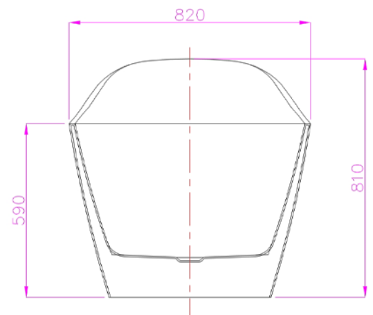
SEZIONE G-G
