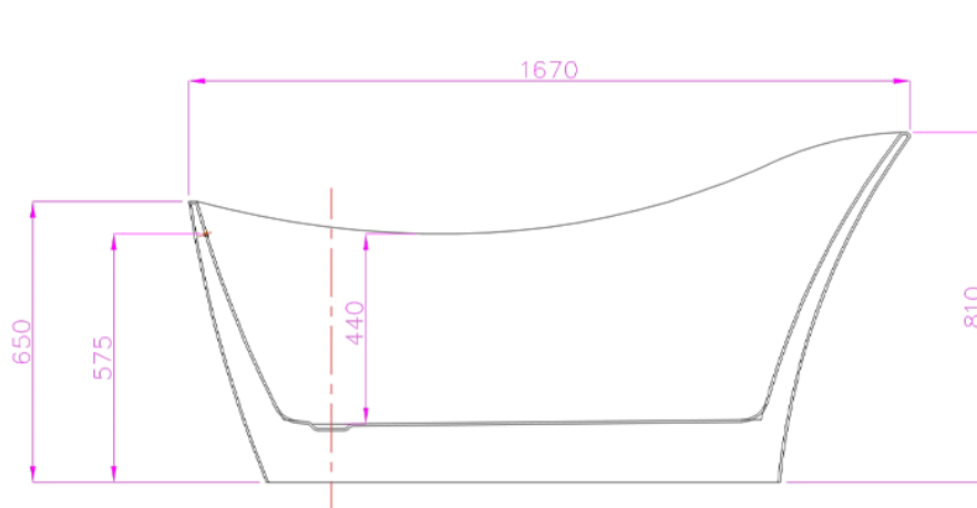
SEZIONE F-F
