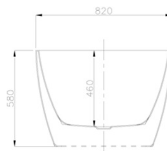
SEZIONE G-G
