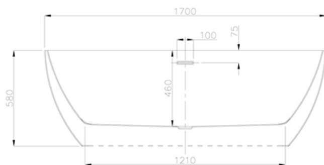
SEZIONE F-F
