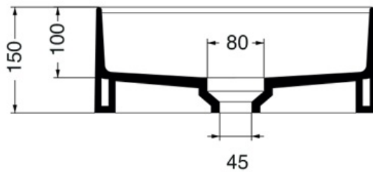
SEZIONE B-B'
